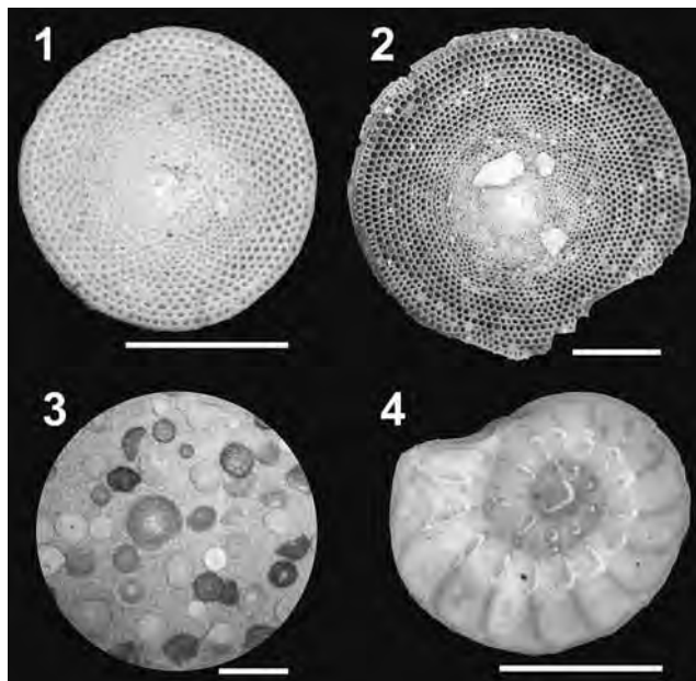
写真1 海浜砂から産する有孔虫殻. 1-3 : Marginopora sp., 4 : Operculina sp. スケールは, 1, 2, 4 が 1 mm を, 3 が 5 mm を示す.
