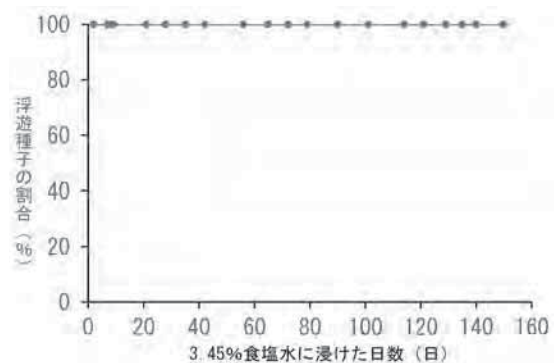
図1 チョウジソウ種子の浮遊能力試験結果
